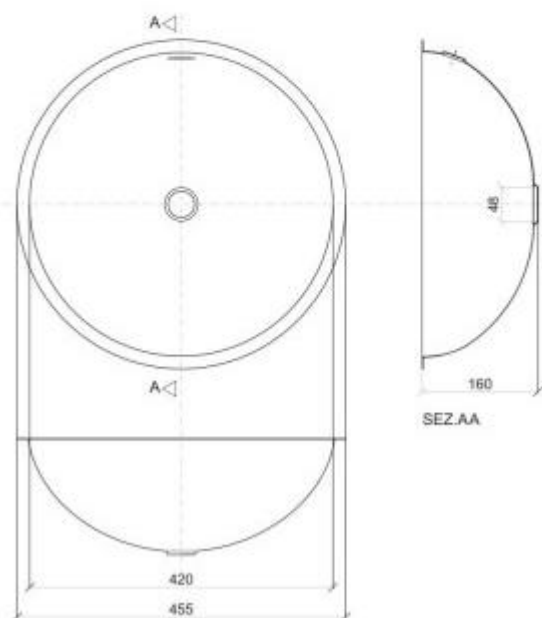
Lavabo rond en acier Ø 455 mm h679_29
